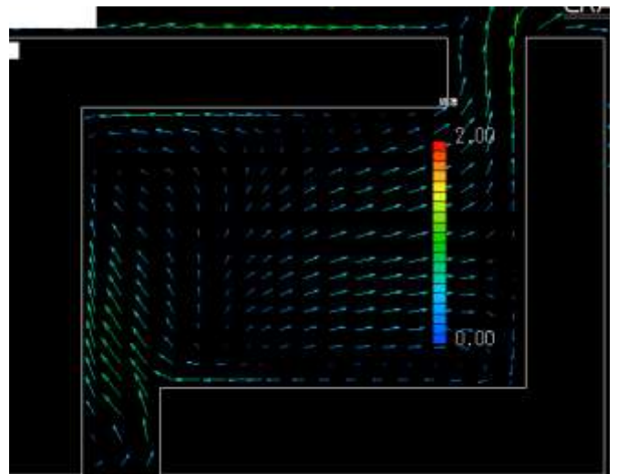
図15 MODEL_Nの囲み型の風速ベクトル(GL+1m)
