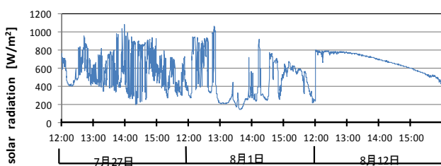
図4 実測日全日程における日射量の比較
