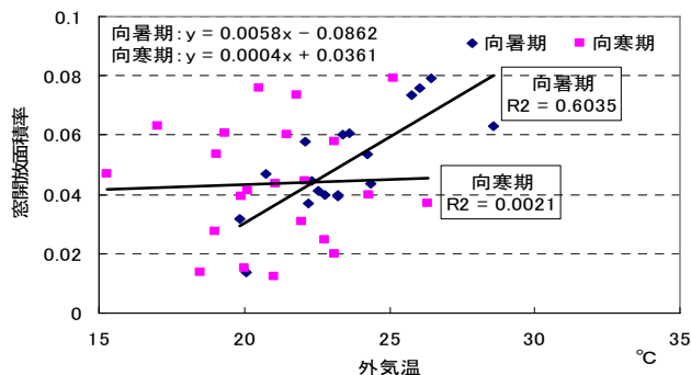
図 4.6 温度感 4 に対する外気温と窓開放面積率
