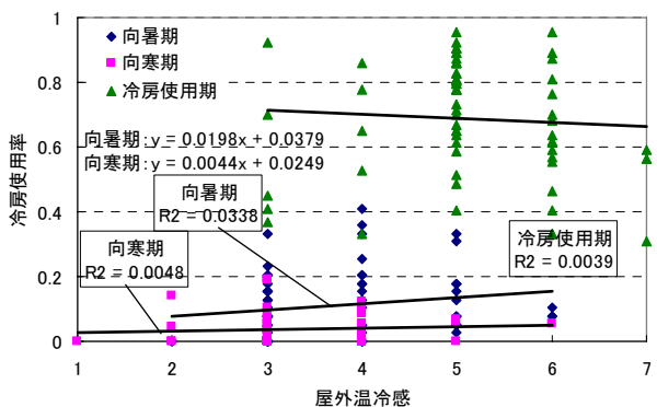
図 4.4 冷房使用期前後の屋外温度感と冷房使用率
