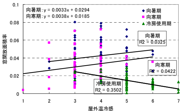
図 4.3 冷房使用期前後の屋外温度感と窓開放面積率
