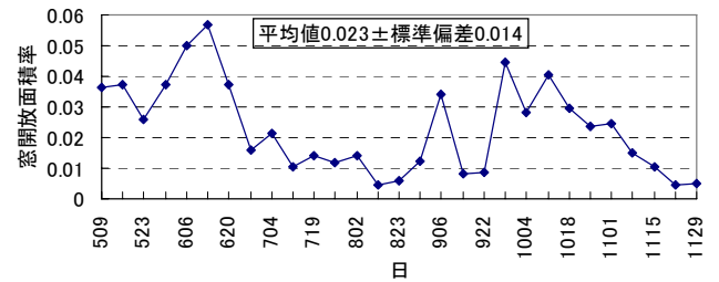
図 3.5 窓開放面積率の推移
