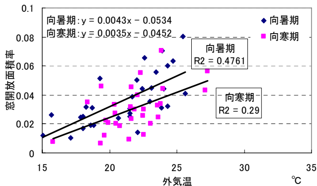
図 4.5 温度感 3 に対する外気温と窓開放面積率
